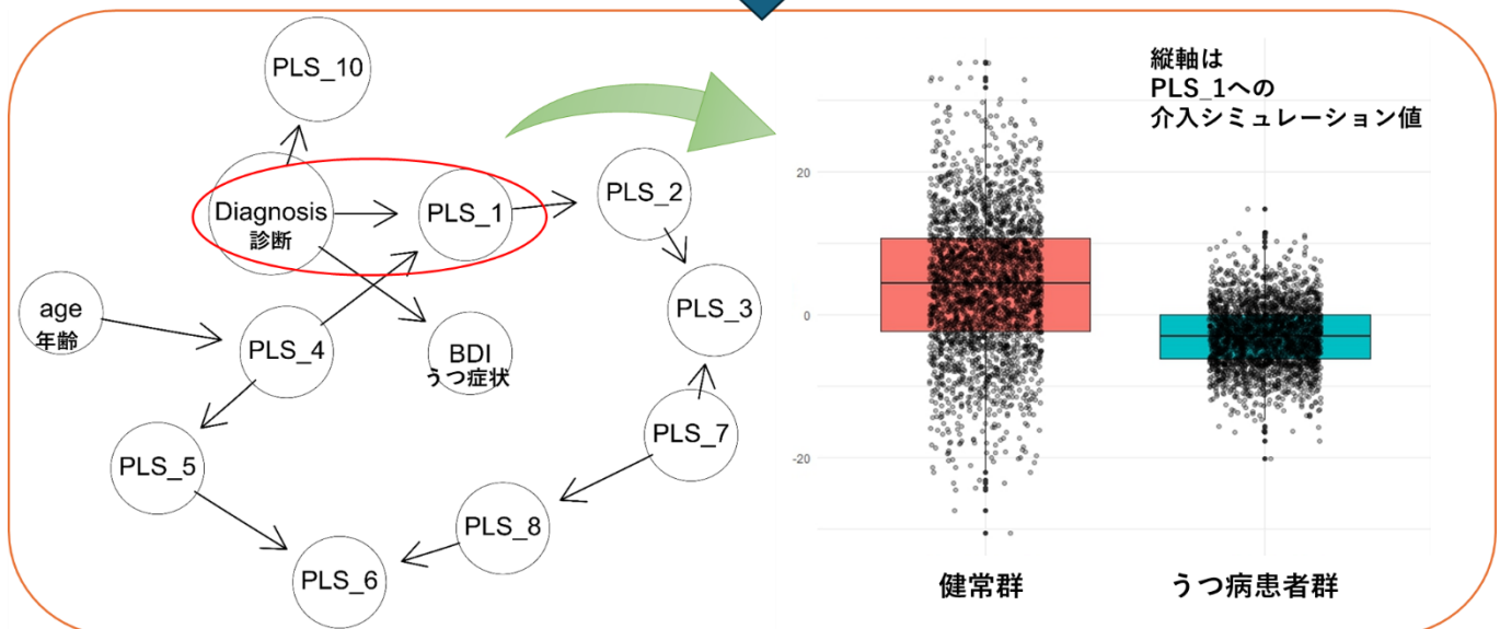
図 ベイジアンネットワークに基づく指標間の関係性（左図）と診断状態を仮定したときの PLS_1 の変化（右図）
